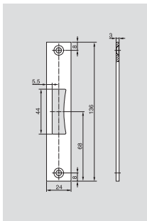
Ответная пластина 74.5 С прямыми углами.
