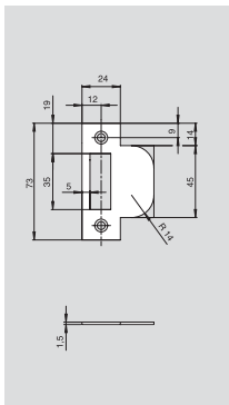
Ответная пластина 23 С прямыми углами.
