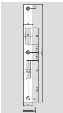
Ответная пластина 71.7 С прямыми углами.
