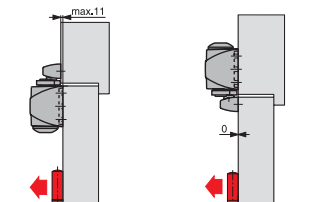
Монтаж на створку двери со стороны петель
