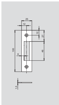
Ответная пластина 21 С прямыми углами.
