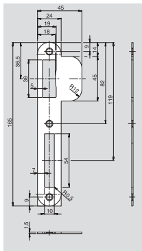
Ответная пластина 20 С прямыми или за- круглёнными углами
