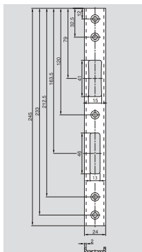
Ответная пластина 71.5 С прямыми углами.
