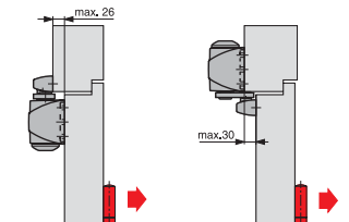
Монтаж на створку со стороны, противоположной петлям
