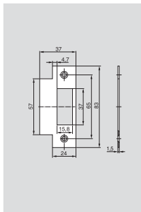
Ответная пластина 75.5 С прямыми углами.
