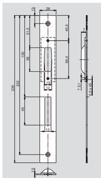
Ответная пластина 27 С прямыми углами.
